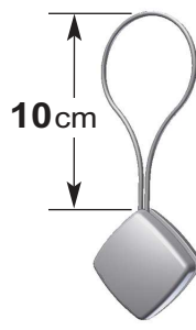
Art.-Nr. 16 CQ quadratisch 28 x 28 mm
